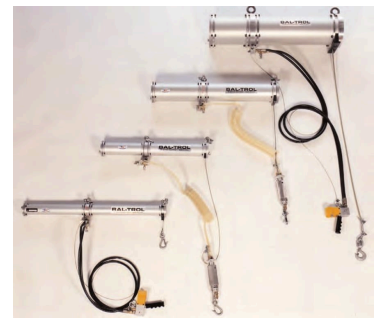
Modular Ratio (M) Dạng module tiết kiệm không gian, tải lớn nhất tới 363 kg (M-40), hành trình 0,3–4,5 m.
