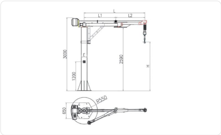
Bản vẽ kích thước cần khớp nối cân bằng phía sau
