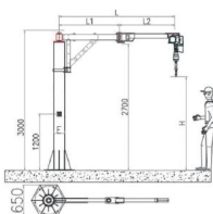
Bản vẽ kích thước cần cân bằng khớp nối phía trước
