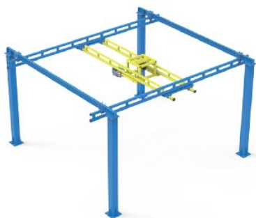
Kiểu Khung Dầm Đôi Với Chiều Cao Móc Tối Đa
