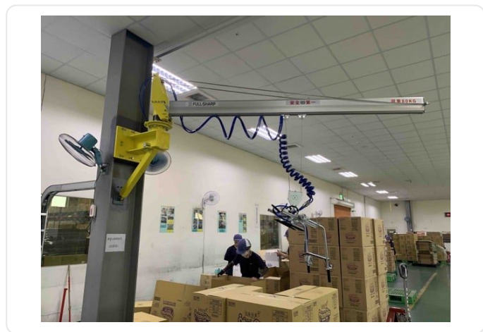
Gắn lên cột Wall mounted
