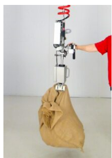
Kẹp tổ hợp bao tải & thùng carton Giác hút · bao tải & carton đa kích cỡ
