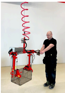
Kẹp tổ hợp cho thùng hộp (giác hút + móc)
