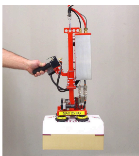
Kẹp tổ hợp thùng hộp & xô Cơ học · thùng hộp & xô · đổi cơ cấu
