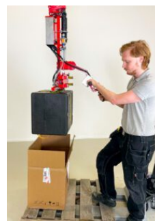
Kẹp tổ hợp cho quạt thông gió Cơ học + Giác hút · đóng gói, xếp pallet
