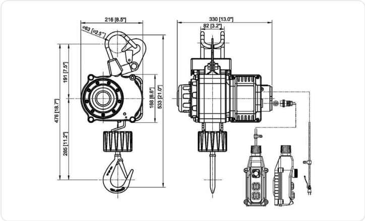
Kích thước CSH-250
