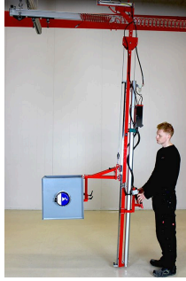
Manhattan Combi-Gripper 89-11763 Cơ khí + chân không · bộ trao đổi nhiệt, mô-tơ
