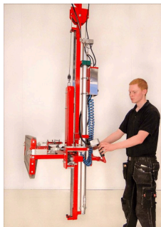
Manhattan đầu nâng khối đá Nâng & xoay khối đá · tải 50 kg
