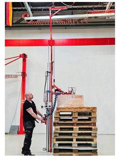
Manhattan nâng cuộn có camera Cuộn thép, giấy, dây, nhựa · camera định vị
