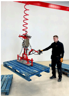
Manhattan đầu nâng pallet Nâng & xếp chồng pallet · tải 45 kg
