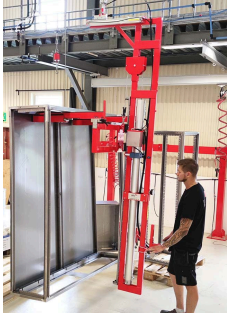
Manhattan nâng thùng carton lớn Giác hút · hành trình 2.1 m · ngành nội thất
