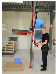
Manhattan nâng thùng carton Giác hút · không gian nhỏ · thay thế xe nâng
