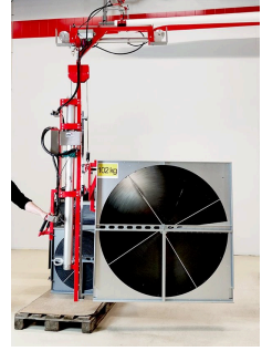
Manhattan combi cho rotor Cơ khí nâng rotor + hút chân không nâng tấm KL
