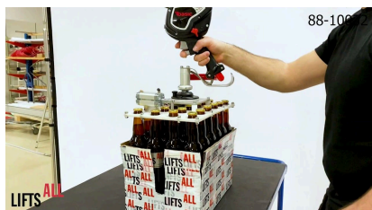
Kẹp chai cơ Bản 88-10063 / 88-10032 Dụng cụ nâng lý tưởng cho nhà máy bia – kẹp và nâng kết chai an toàn, công thái học. Kết chai · Nhà máy bia · Mã: 88-10063
