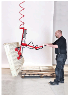
Kẹp khung giường 89-12031 Dùng trong ngành nội thất để nâng và nghiêng khung giường. Tải tới 30 kg. Tải: 30 kg · Nâng & nghiêng · Mã: 89-12031
