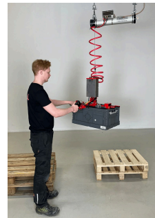
Kẹp hộp nhựa 89-12353 Thiết kế nâng hộp/thùng dễ dàng và an toàn tới 25 kg – ngành thực phẩm. Tải: 25 kg · Thực phẩm · Mã: 89-12353
