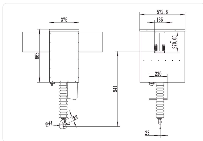
Bản vẽ kích thước Clean Room Travelling Type
