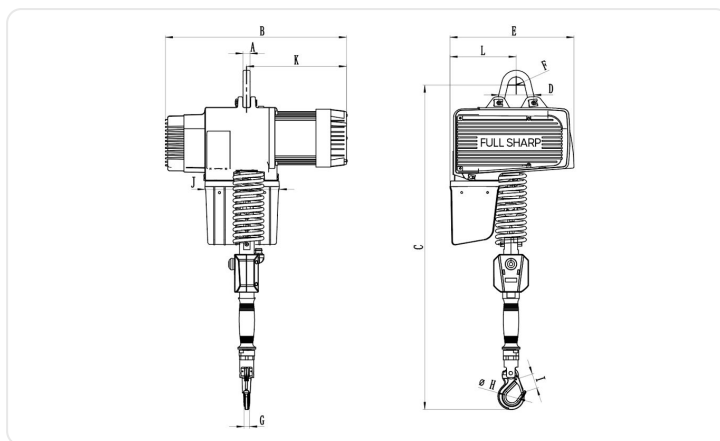
Bản vẽ kích thước pa lăng FS-D2L
