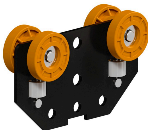
Con Chạy Tải — Ray RAD6110 Tải tối đa 1.600 lbs [725 kg] MRTA6106 6 lbs [2,72 kg] RAD6110
