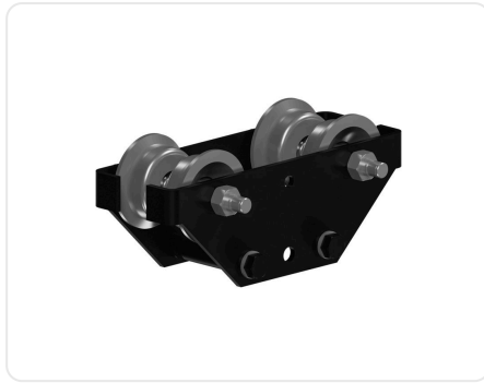
Con Chạy Dầm W / I-Beam Tải tối đa 3.000 lbs [1.360 kg] RTA2013 23 lbs [10,4 kg] W-Beam · I-Beam
