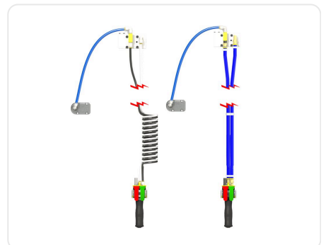
Pendant Tandem Lên/Xuống Dùng cho palăng cân bằng Tandem BCS2326 / BCS3330 Ống xoắn / thẳng Tandem
