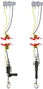
Tay Điều Khiển Feather-Touch Tay ngang / tay đứng BCS2213 / BCS2214 12,4 lbs [5,64 kg] 100lbs
