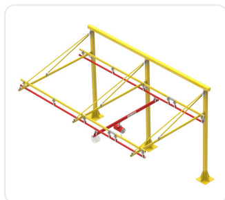
Kết cấu khung một bên chân
