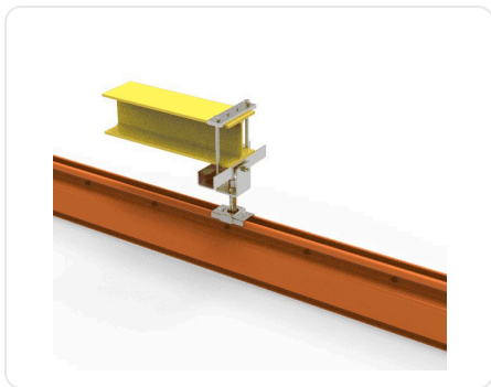
Bộ treo thanh ray dọc
