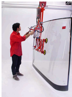
Nâng kính chắn gió 89-11857 Một người mang được tấm kính 100 kg. Hỗ trợ mang, nghiêng và xoay tấm kính, kẹp chắc chắn. Tải: 100 kg · Nghiêng & xoay · Kính chắn gió · Mã: 89-11857
