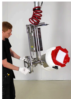
Kẹp phuy & thùng bia 89-10911 Nâng, nghiêng và xoay phuy, thùng bia tới 30 kg. Chế tạo riêng cho phòng sạch. Tải: 30 kg · Nghiêng & xoay · Phòng sạch · Mã: 89-10911
