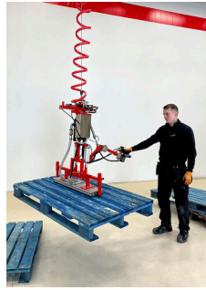
Kẹp Pallet 89-12178 Một dụng cụ nâng pallet, nắp pallet và khung viền pallet. Tải 45 kg, điều khiển PSH. Tải: 45 kg · Pallet/nắp/viên · PSH · Mã: 89-12178
