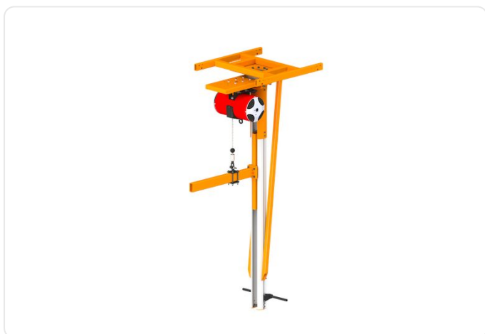
ATA4000 - trụ tròn (Round mast)
