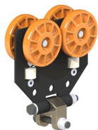
Xe trượt tải có ách - RAD7510 Tải tối đa: 3.000 lbs [1.360 kg] MRTA7723
