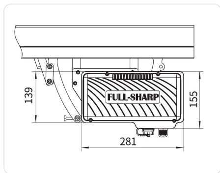
Bản vẽ kích thước (1)
