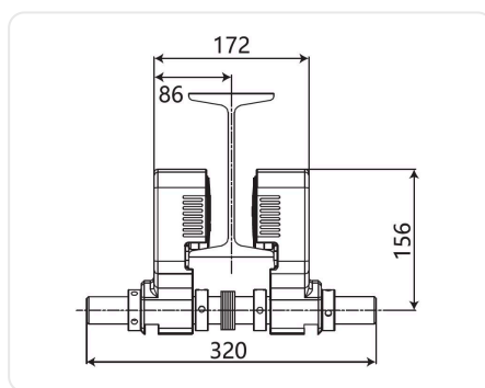
Bản vẽ kích thước
