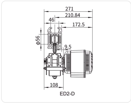
FS-ED2-E Bản vẽ kích thước
