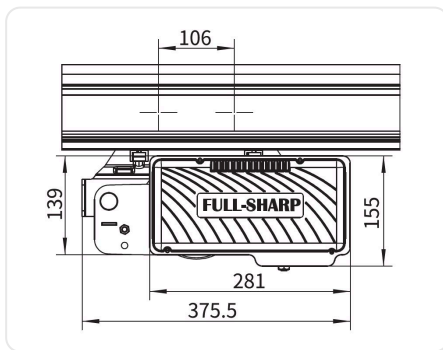
FS-ED2-D Bản vẽ kích thước
