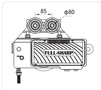
Bản vẽ kích thước (2)
