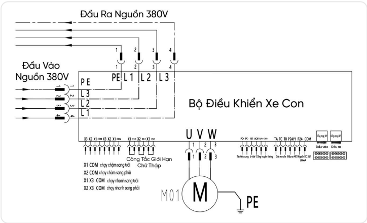
Sơ đồ đấu dây
