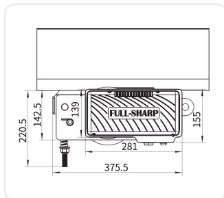
Bản vẽ kích thước (1)
