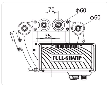
Bản vẽ kích thước (2)
