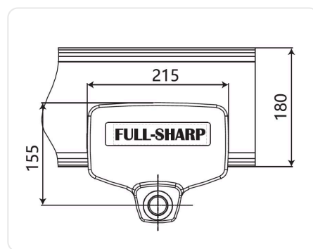
■ Trolley Điện Servo — Ray Thép Chữ I
