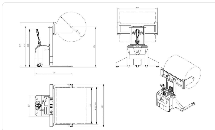
Bản vẽ kích thước xe nâng cuộn nằm ngang
